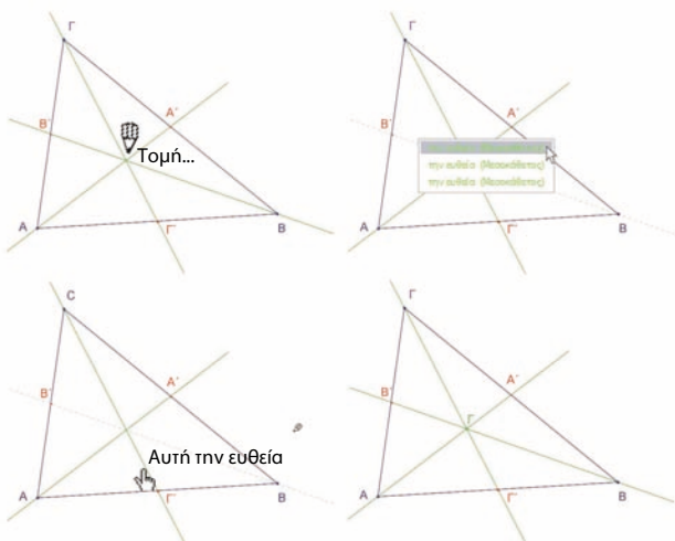
Σχήμα 4.3: Κατασκευή του σημείου τομής των διαμέσων και επίλυση των ασαφειών μιας επιλογής.
