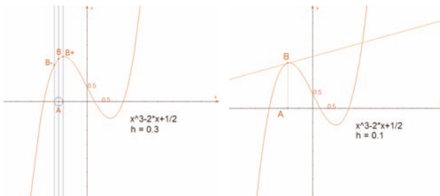
Σχήμα 14.5: [αριστερά] Κατασκευάζονται στην καμπύλη τα τρία σημεία: B- , B , B+ , με τετμημένες: x-h , x και x+h . [δεξιά] Η προσέγγιση της εφαπτομένης στο B , αφού γίνει απόκρυψη των στοιχείων κατασκευής.
