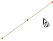
Σχήμα 3.4: Κατασκευή του μέσου ενός τμήματος.
