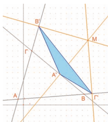
Σχήμα 13.3: Κατασκευή του πλέγματος με τη βοήθεια των προεπιλεγμένων αξόνων του σχήματος. Επαναπροσδιορισμός του M ως ελεύθερο σημείο στο πλέγμα.
