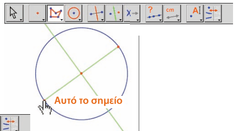
Σχήμα 3.7: Κατασκευή τετραγώνου με έμμεση κατασκευή των σημείων τομής του κύκλου και της μεσοκαθέτου.
