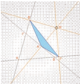
Σχήμα 13.4: Η κατανομή του εμβαδού ενός ποδικού τριγώνου ανάλογα με τη θέση του σημείου M .
