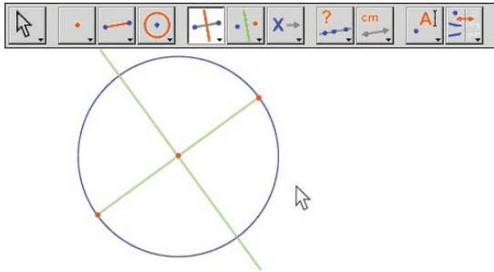
Σχήμα 3.6: Κατασκευή της μεσοκαθέτου ενός ευθύγραμμου τμήματος, για τον καθορισμό της άλλης διαγωνίου του τετραγώνου.
