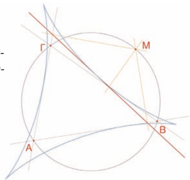
Σχήμα 13.5: Η περιβάλλουσα των ευθειών Simson τριγώνου AB\Gamma ονομάζεται δελτοειδές. Έχει την ίδια συμμετρία με ένα ισόπλευρο τρίγωνο.
